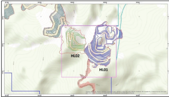
Desain Pit HL01 dan HL02
